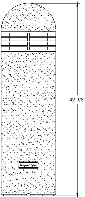
ELEVATION
