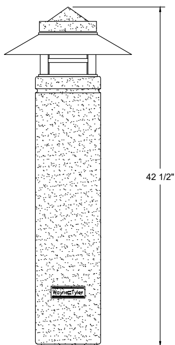
ELEVATION
