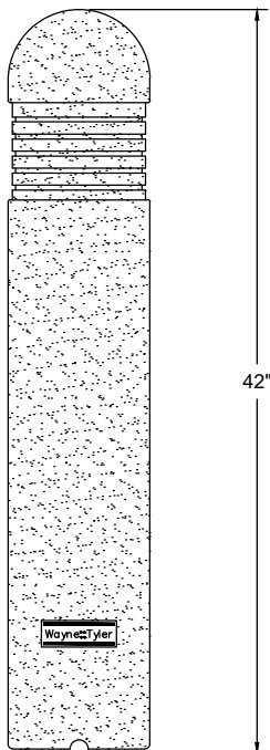
ELEVATION
