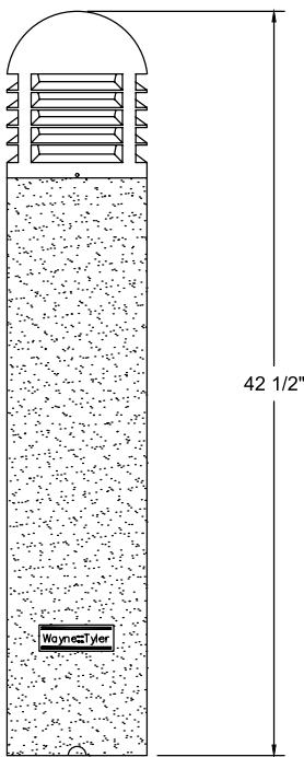
ELEVATION
