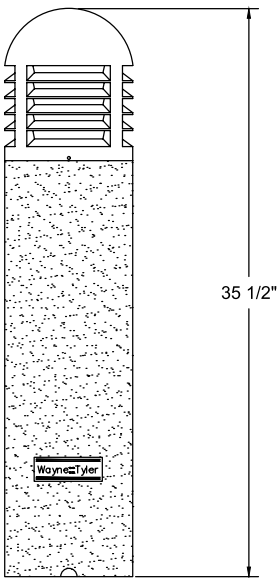
ELEVATION
